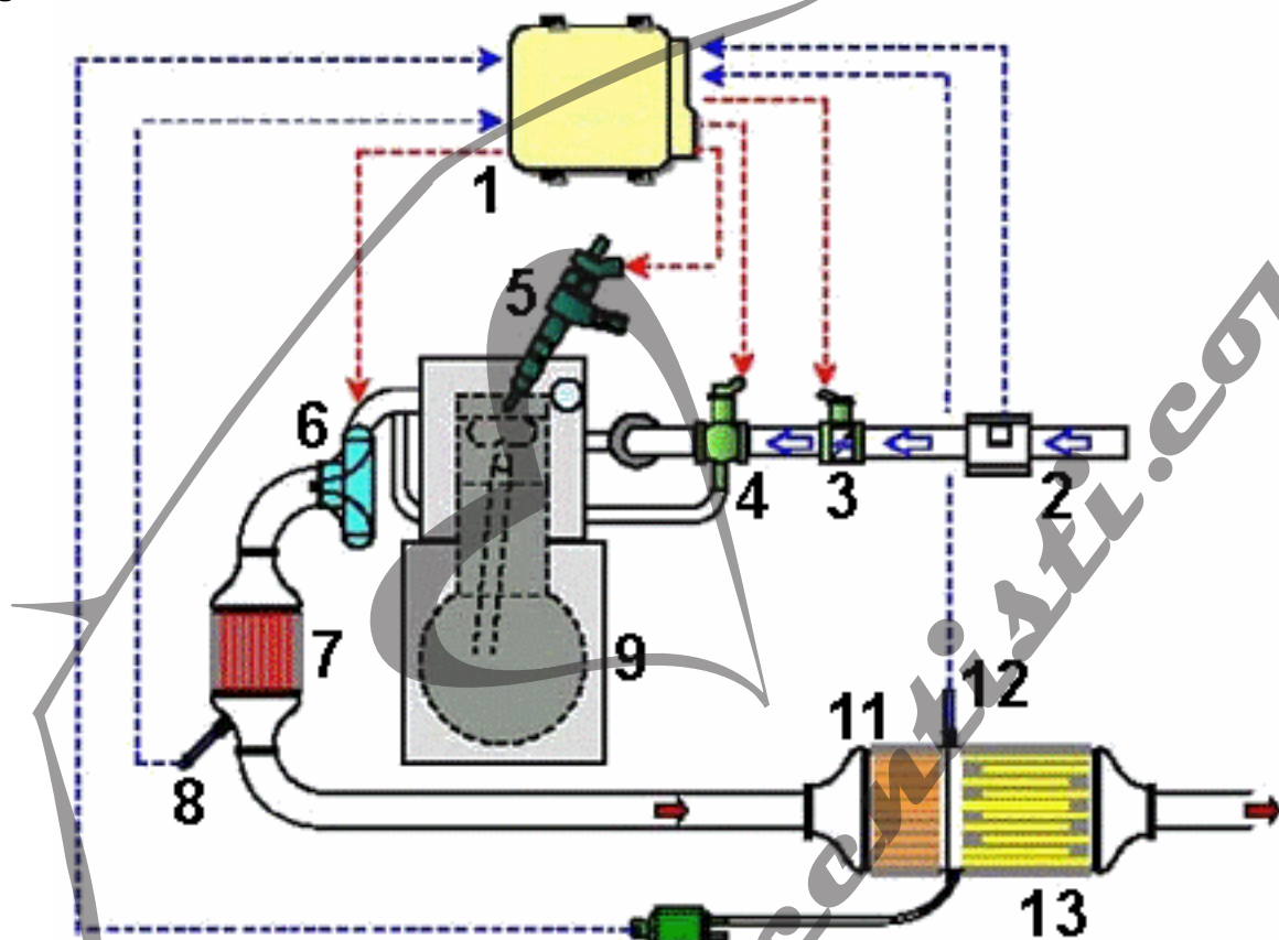
Fig. 5 - Schema Euro 4
