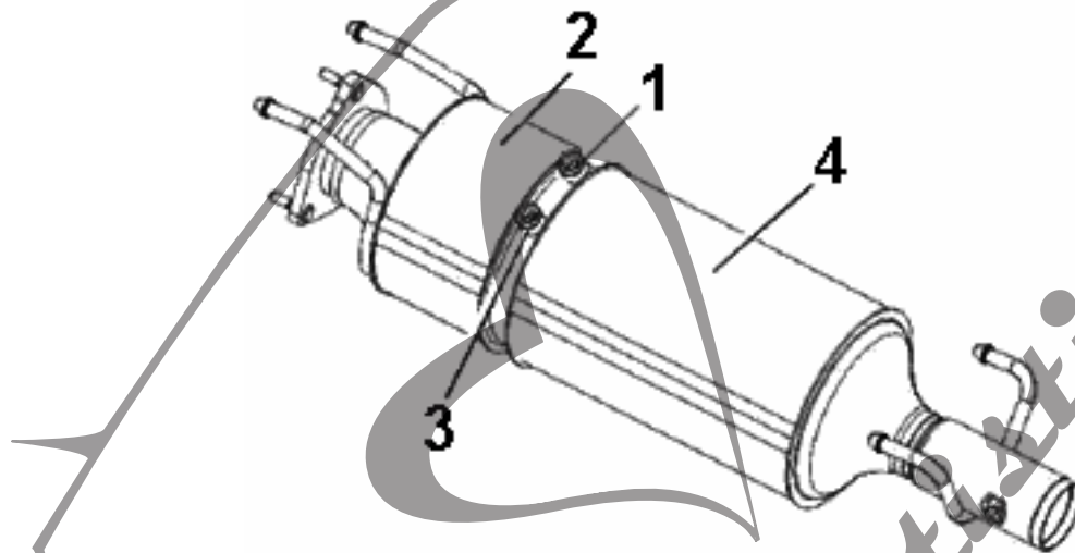
Fig. 7 – Filtro DPF
