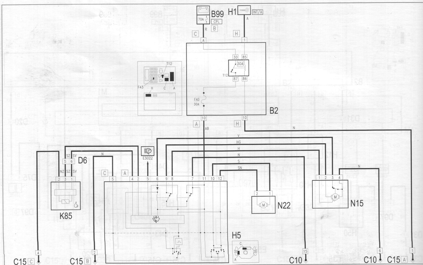
Tergi-cristalli - Lava-cristalli (parabrezza)
